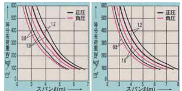
単純梁
