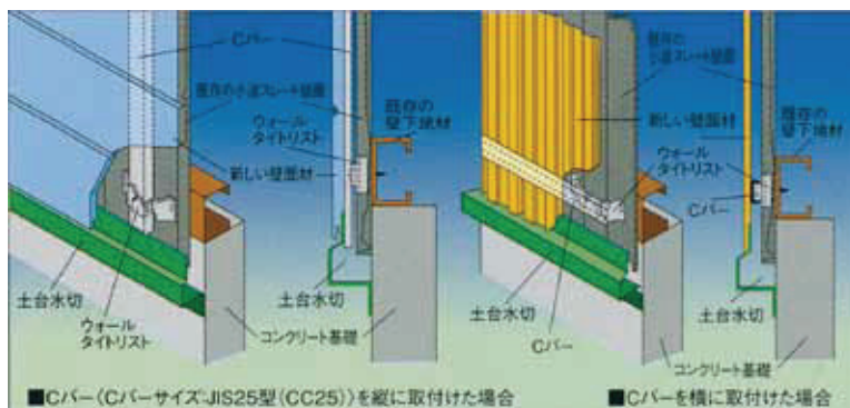
タイプ2 ストレート小波一般部用(外壁) 亜鉛めっき鋼板
