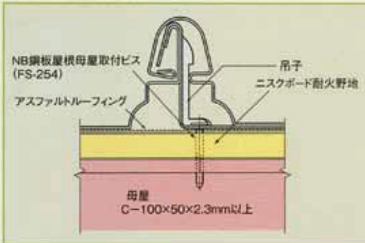
縦着屋根吊子取付け参考図
